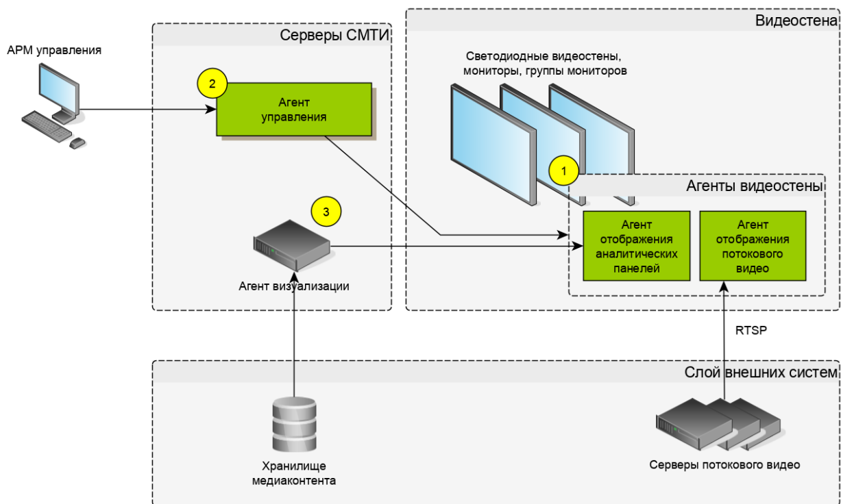
Рисунок 1. Схема взаимодействия компонентов СМТИ, включая модуль визуализации в виде агентов видеостены
